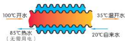
图2 第三代热交换器节能原理图
